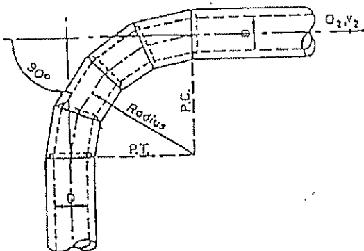
CASE VII CONDUIT ON 90° CURVES †
